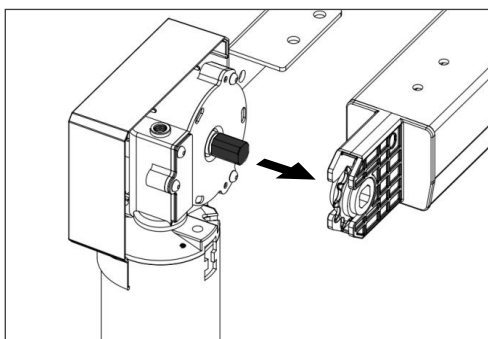
3 • Coloque el motor en la guía insertando el eje de salida en el encaje hexagonal del canal.
