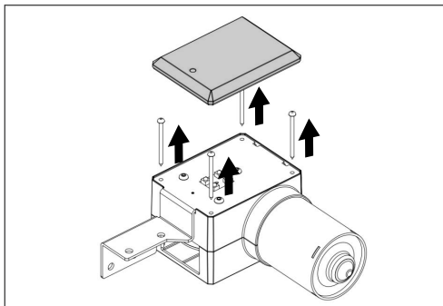
1 • Retire la tapa del motor y afloje los tornillos.
