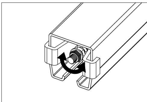
5 • Ajuste la tensión de la cadena apretando o aflojando la tuerca.
