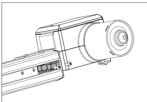
6 • Cuando terminar, coloque los tornillos de fijación.
