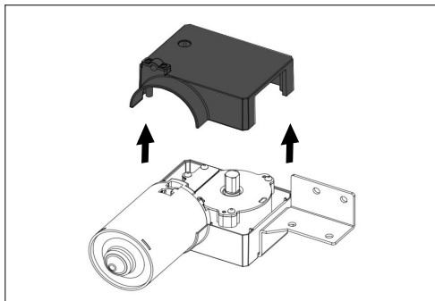
2 • Gire el motor en sentido contrario y ábralo tirando de la carcasa hacia arriba.
