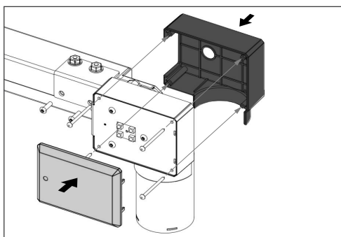
4 • Vuelva a cerrar el motor de nuevo montando la tapa y la carcasa.
