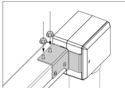
7 • Apriete los tornillos de fijación del motor a la placa.
